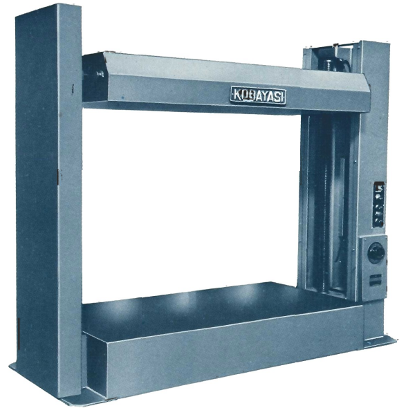
■ KF-P 357型 (標準式)
